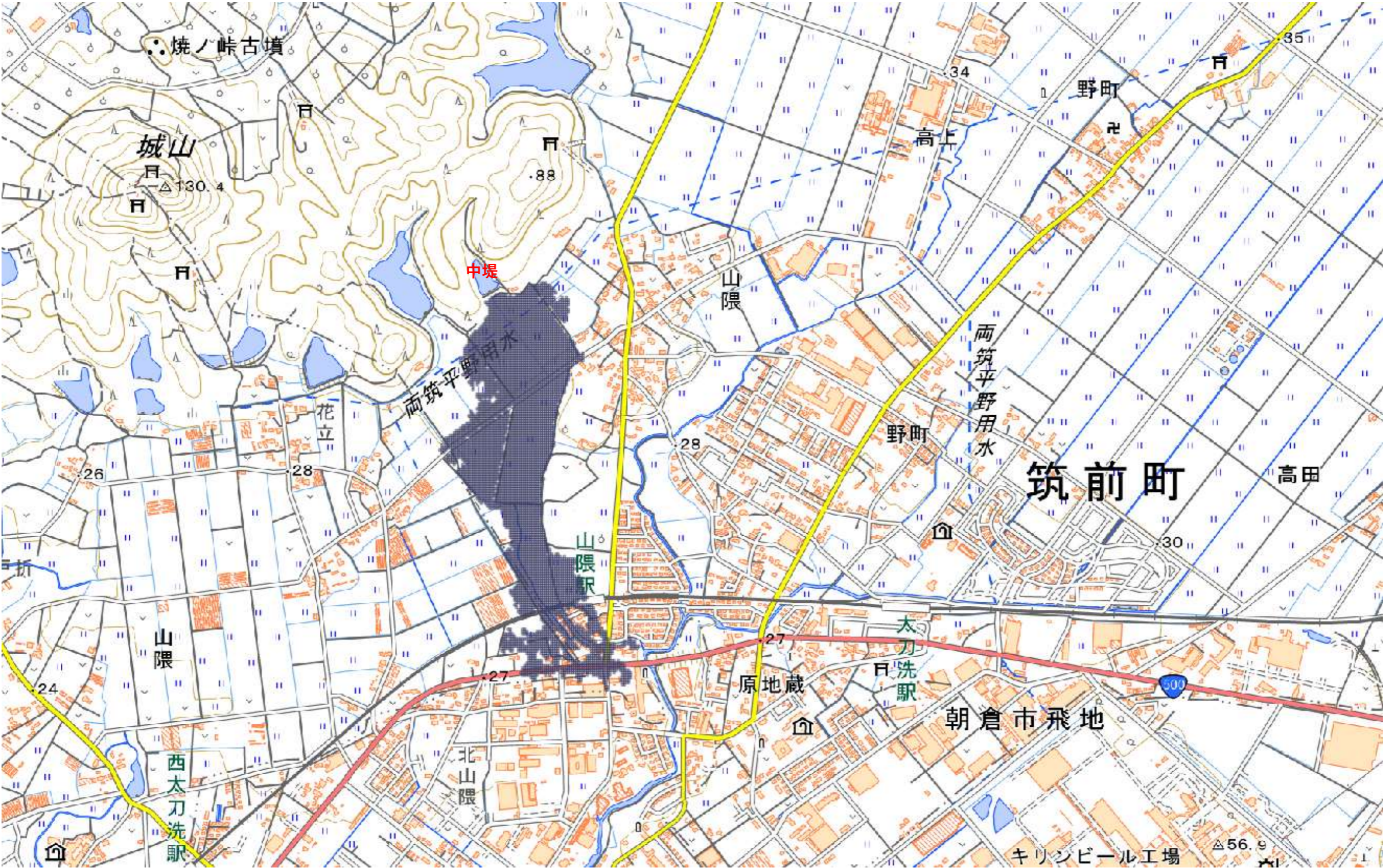
筑前町(中堤)の想定浸水区域図
