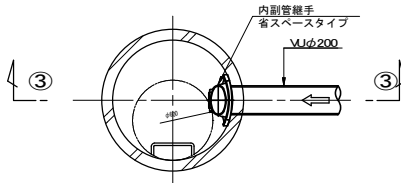
平面図
