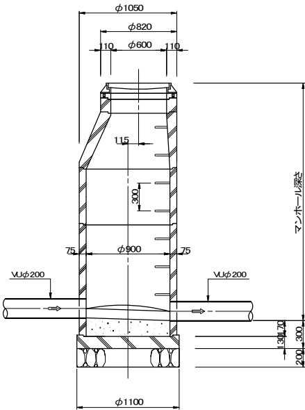
①—①断面図
