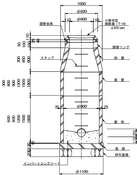
②—②断面図
