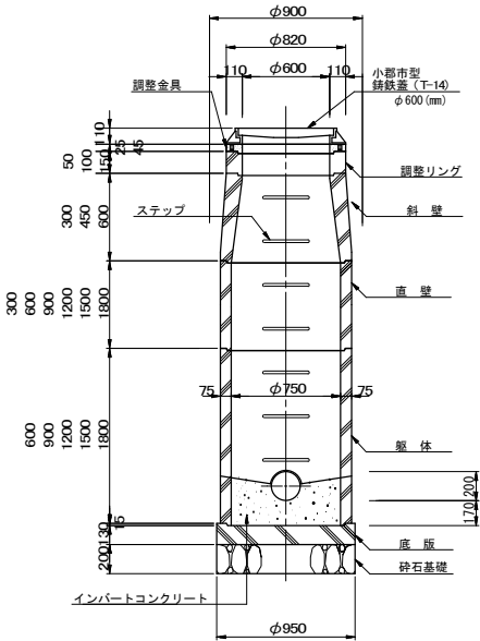
②—②断面図
