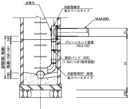
③—③断面図
