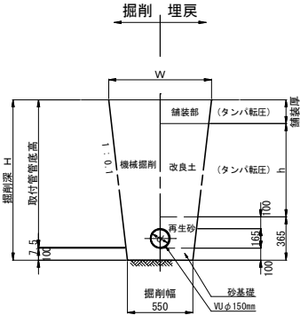
タイプ-1 (素掘)
