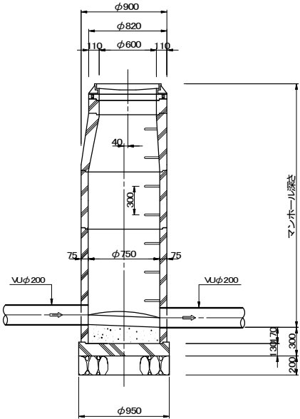
①—①断面図
