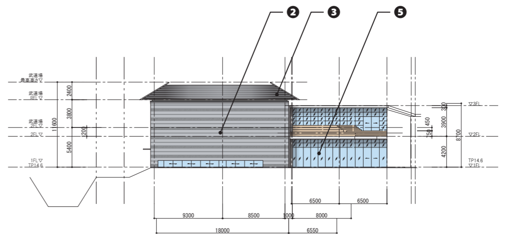
武道場 南立面図
