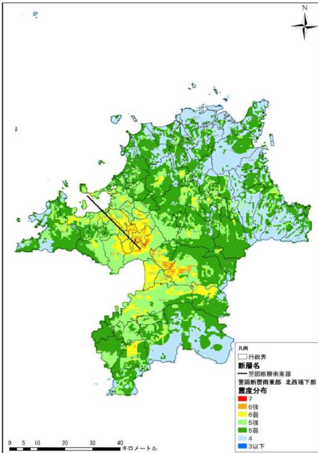
震度分布図 — 警固断層（南東部）（破壊開始：北西下部） —
