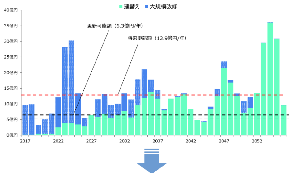
図 長寿命化を実施する前（上）と実施した場合（下）の建築物の更新費
