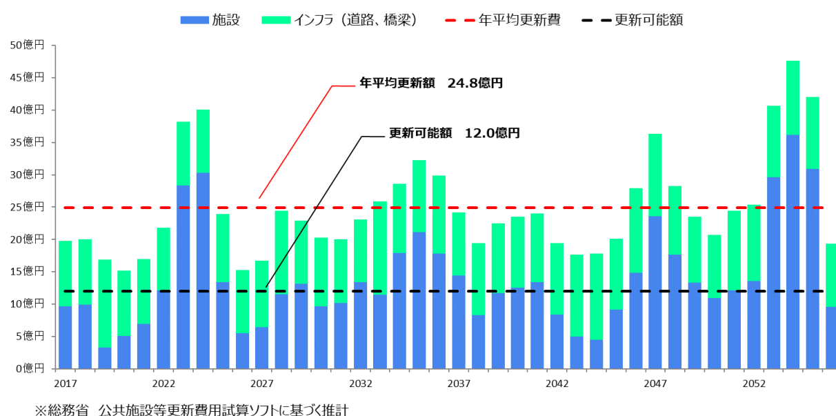
図 公共施設等（建築物、道路、橋梁）の年度別将来更新費（2017 年度から 2056 年度）
